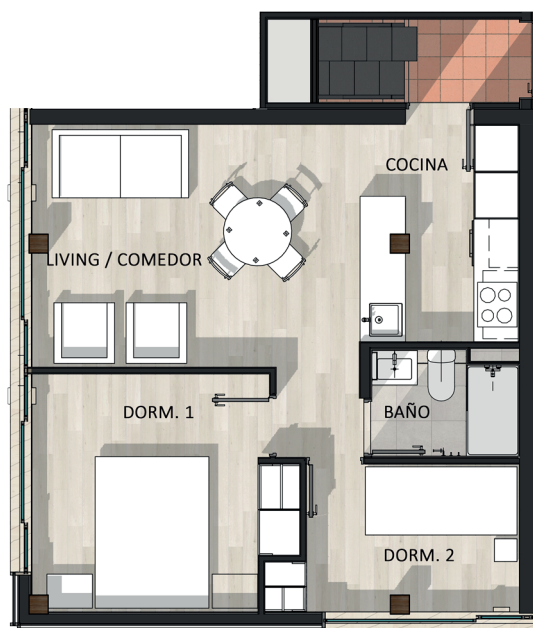
PLANTA PISO 3
