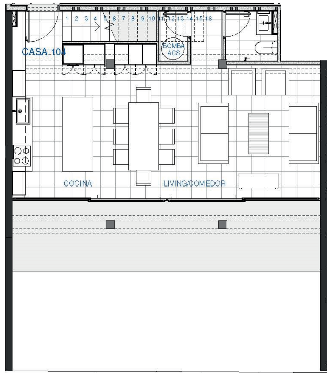
PLANTA PISO 1
