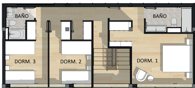
CASA 02, PISO 2
